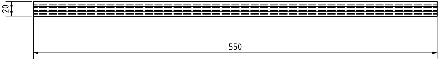
VIEW2 ( 2 : 1 )
